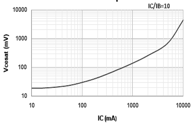
Vcesat Vs. Ic plot
