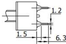
PC terminal(2)
