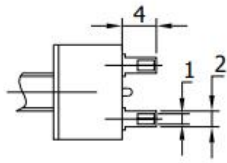
Soleer terminal(1)
