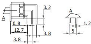
PC-V terminal(4)
