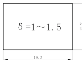
安装面板尺寸 PANEL CUT-OUT
