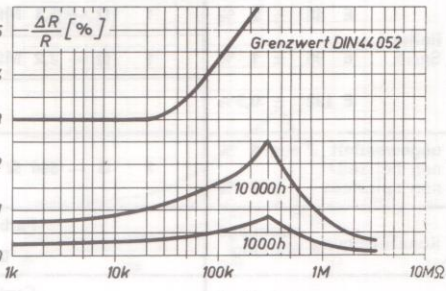
Belastung Endurance + 70°C 1000 h Load life
