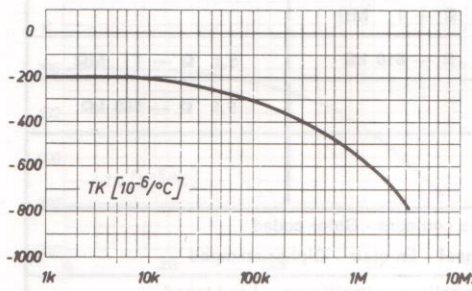
Temperaturkoeffizient Coefficient de température Temperature coefficient
