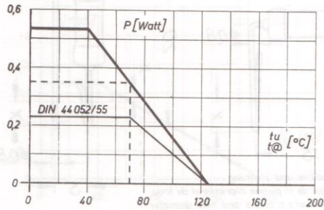
Lastminderung Derating
