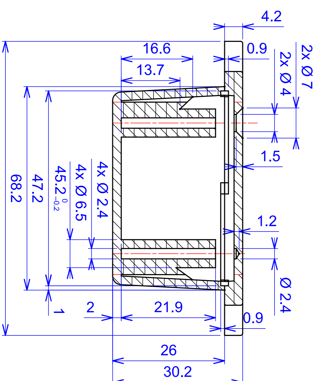
B-B
