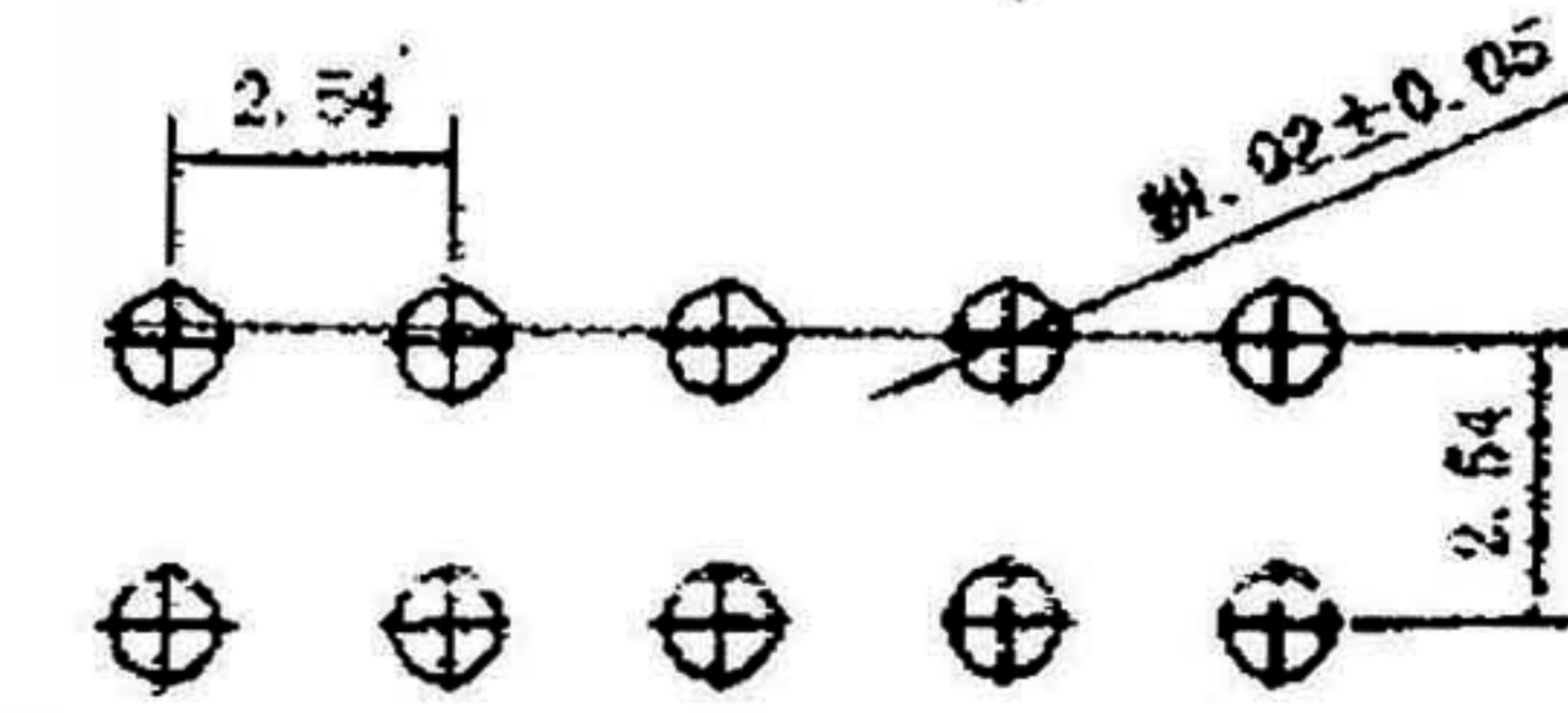
P.C.B. Hole Layout
