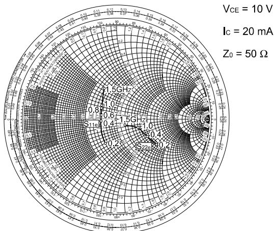
S-PARAMETER
